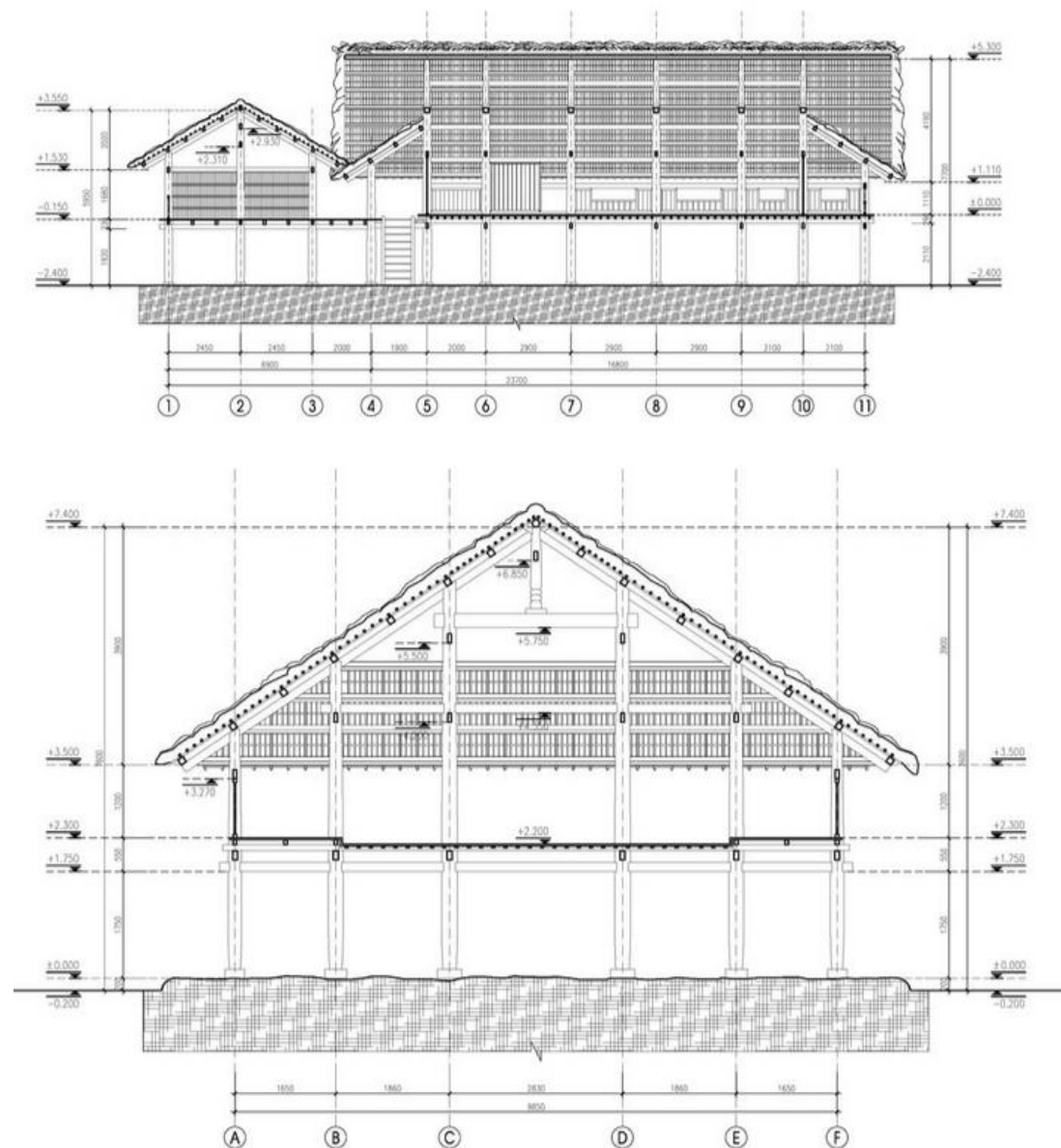
MẶT CẮT 1-1
