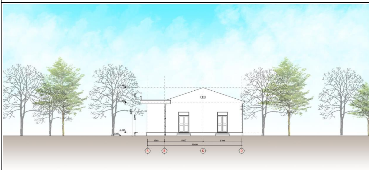
Mặt bên trục A-D
