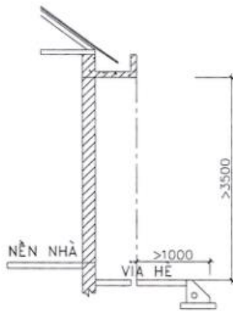
a) Trường hợp phần đưa ra là sê nô, ô văng và mái dốc
