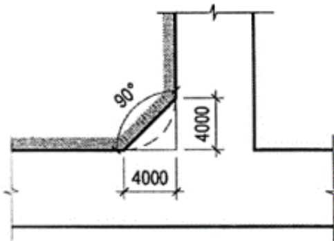
c. Kích thước vạt góc tại góc cắt giao nhau 90^\circ
