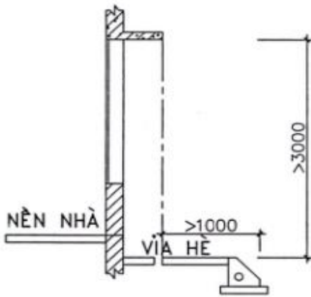
c) Trường hợp phần đưa ra là ô văng
