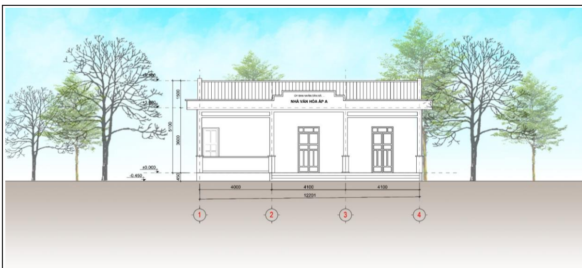
Mặt đứng trực 1-4
