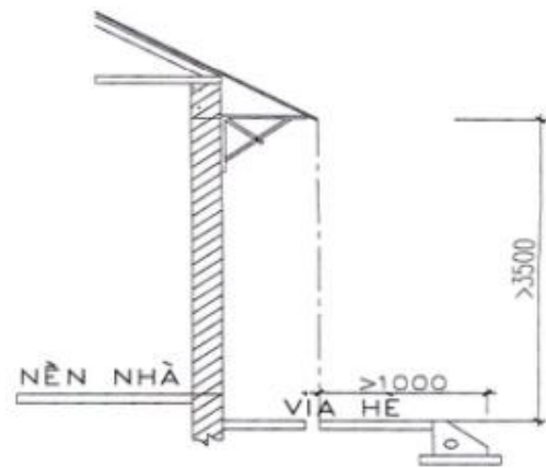
d) Trường hợp phần đưa ra là con sơn mái dốc
