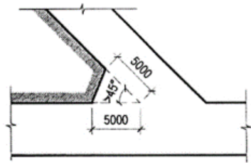
b. Kích thước vạt góc tại góc cắt giao nhau \geq 45^\circ
