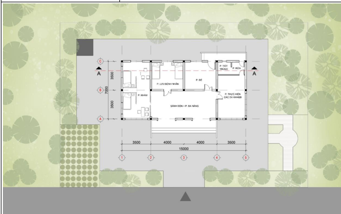
Mặt bằng
